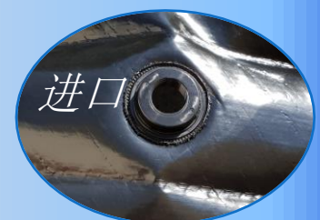
一体化的1/2"内螺纹
